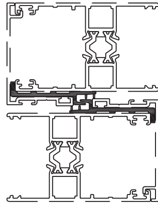
RTC-40 Aro móvel p/ folhas eleváveis
